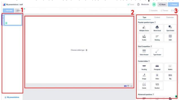
Fig. 4: Pantalla principal.
